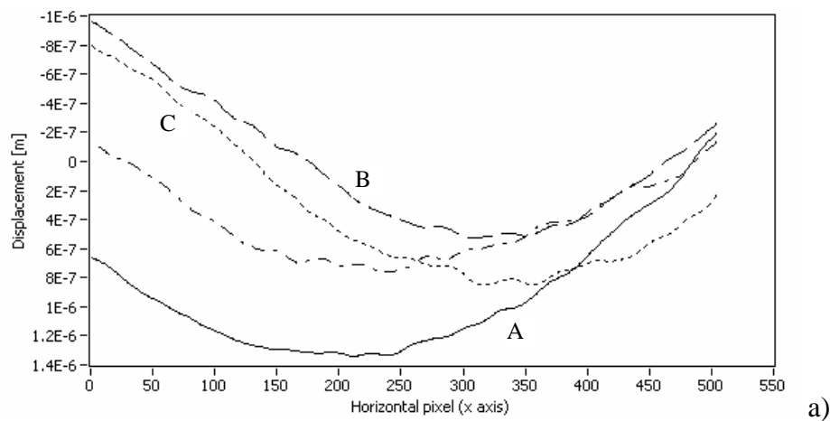
Figure 6 – Analisi dello spostamento nella configurazione I per il provino in Abete rosso: a) spostamento u vs pixel orizzontali; b) spostamento u vs pixel verticali
