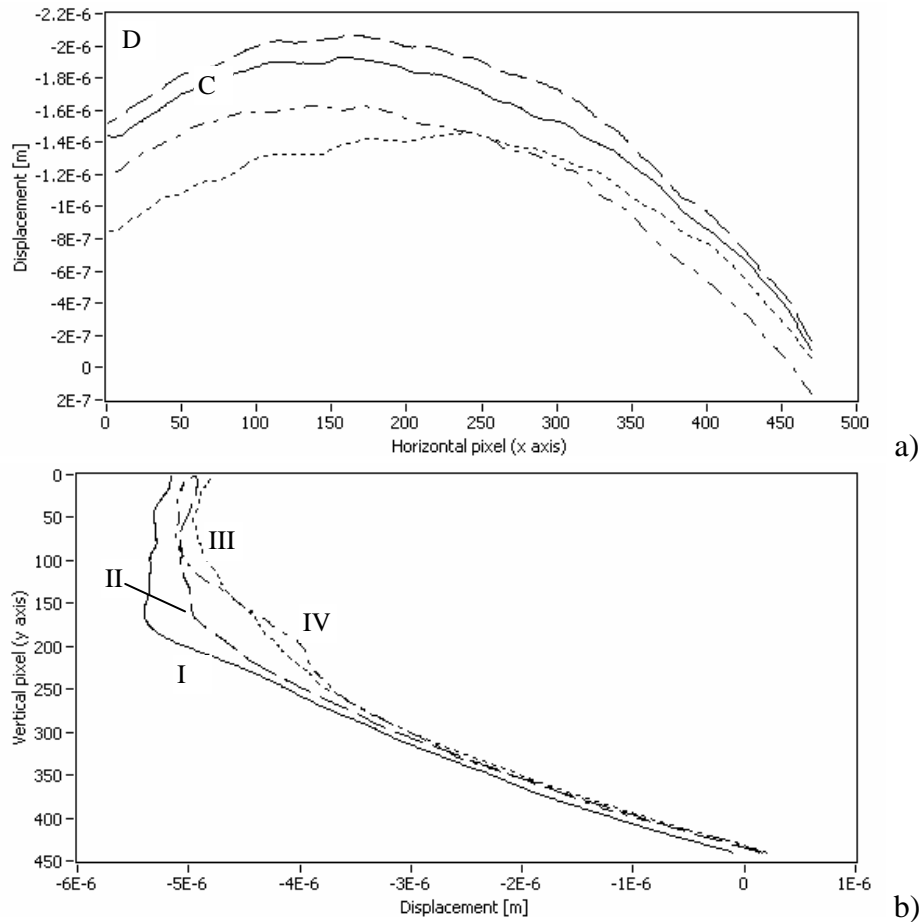
Figure 9 – Analisi dello spostamento nella configurazione II per il provino in Ciliegio: a) spostamento v vs pixel orizzontali; b) spostamento v vs pixel verticali
