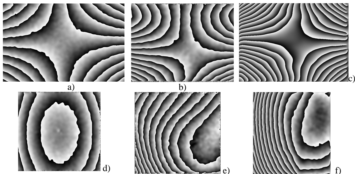
Figure 3 – Campi di frange: a) Plexiglas configurazione I); b) Abete rosso configurazione I); c) Ciliegio configurazione I); d) Plexiglas configurazione II); e) Abete rosso configurazione II); c) Ciliegio configurazione II).
